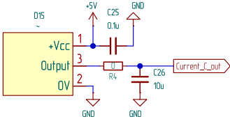
Датчик тока фазы С
