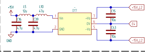
Питание драйвера верхнего ключа фазы В
