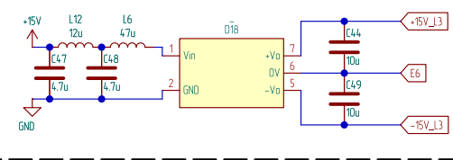
Питание драйвера верхнего ключа фазы С
