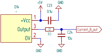
Датчик тока фазы В
