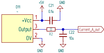
Датчик тока фазы А
